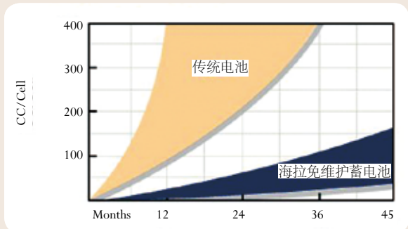
海拉蓄电池与传统电池的水耗比较
