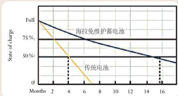
海拉蓄电池与传统电池的自放电比较(25°C)
