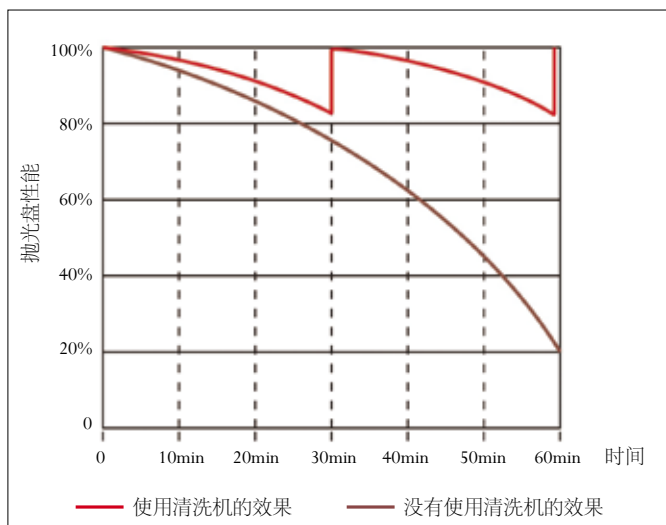
图1 使用/不使用抛光盘清洗机的情况下抛光盘的性能对比
